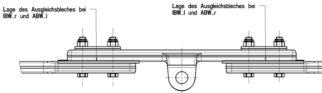
Bild 6 Ausgleich des Versatzes der Zungenbohrungen bei Bogenweichen
