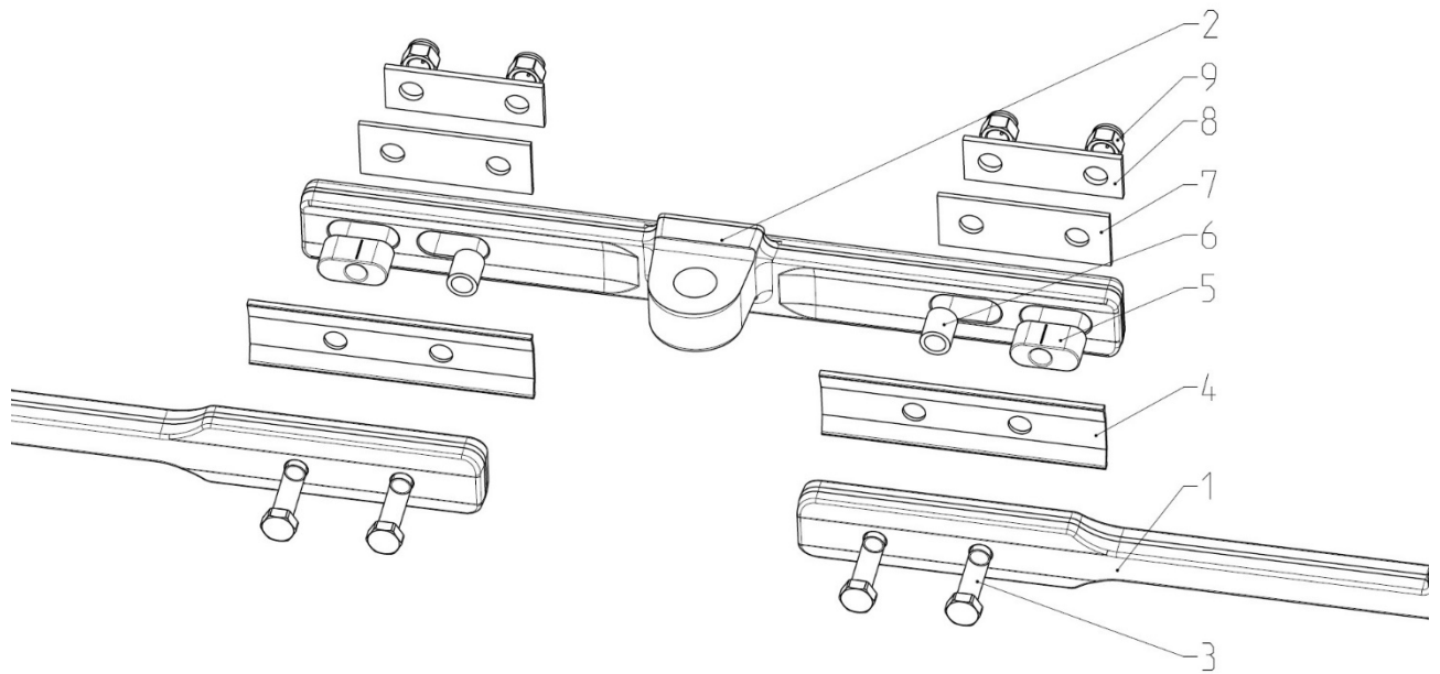
Bild 1 Montage der Schieberstange System UniBar
