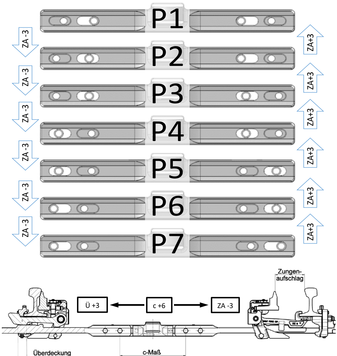
Bild 5 Einfluss der Steckposition auf Zungenaufschlag und Überdeckung
