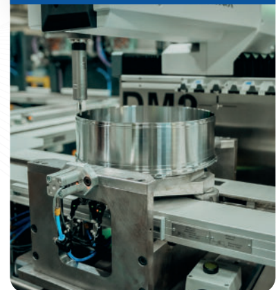
Mechanische Bearbeitung
