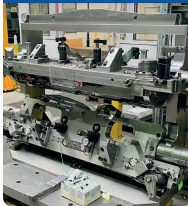
Vorrichtungen
